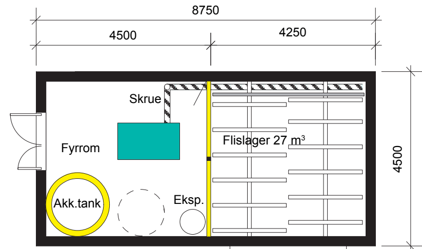
Fyrrom med akkumuleringstank og flislager med stangmater (mot en side)
