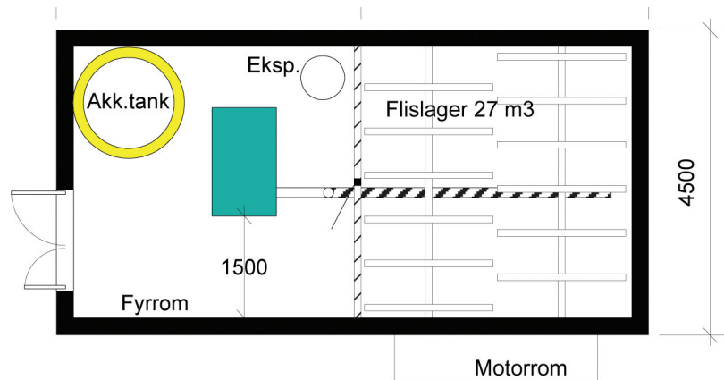
Fyrrom med akkumuleringstank og flislager med stangmater (mot midten)
