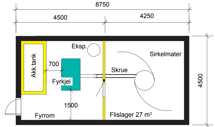
Fyrrom med akkumuleringstank og flislager med sirkelmater
